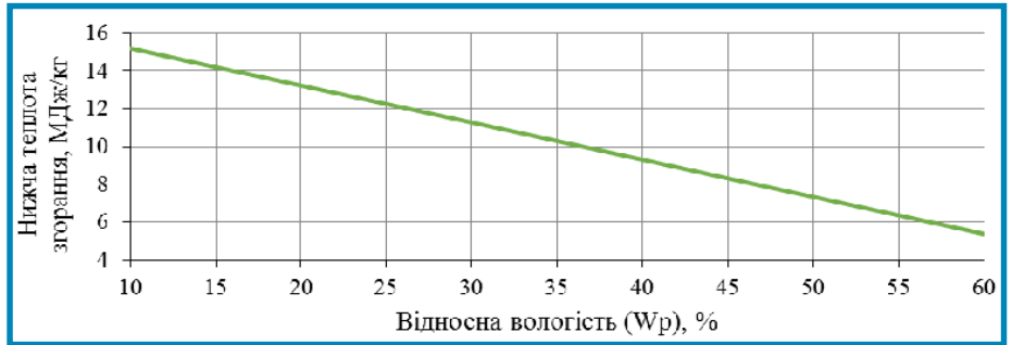
Рис. 3 Графік залежності нижчої теплоти згорання від відносної вологості кукурудзяної соломи.
